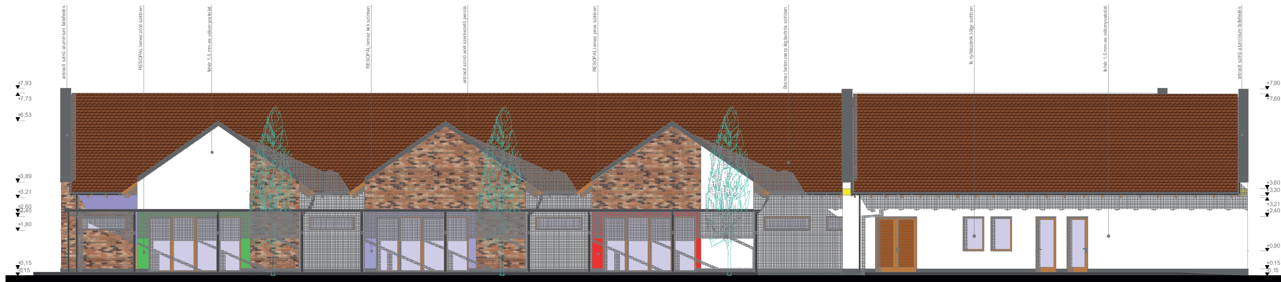
Dél-keleti homlokzat M=1:100
